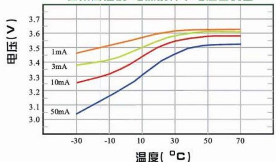
在不同温度,电流条件下电压曲线图
