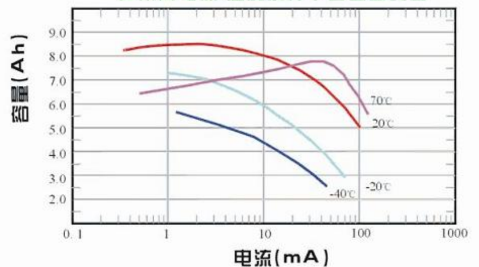
在不同电流,温度条件下容量曲线图
