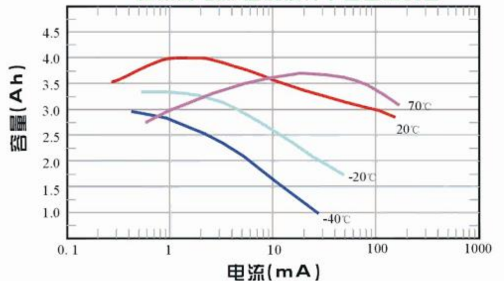
在不同电流,温度条件下容量曲线图
