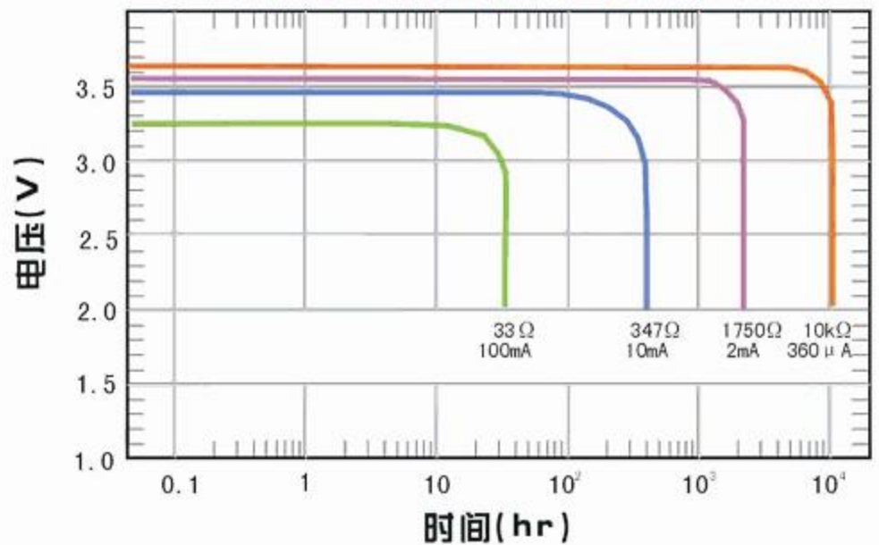
在 23\pm 2^{\circ}\text{C} 条件下放电曲线图
