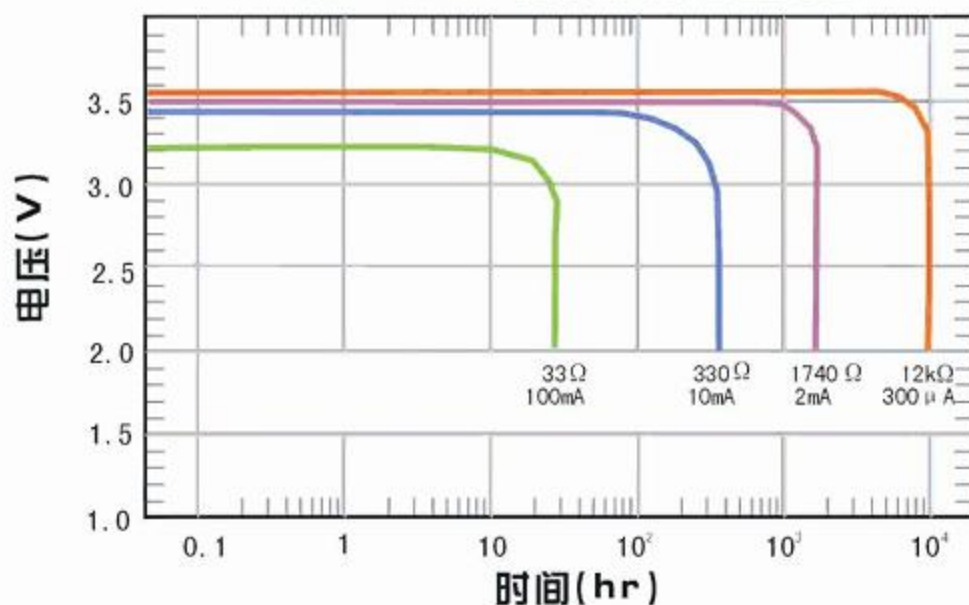
在 23±2 °C 条件下放电曲线图
