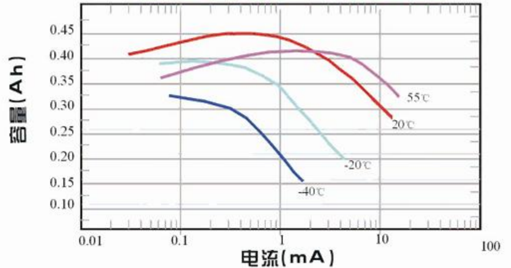
在不同电流,温度条件下容量曲线图
