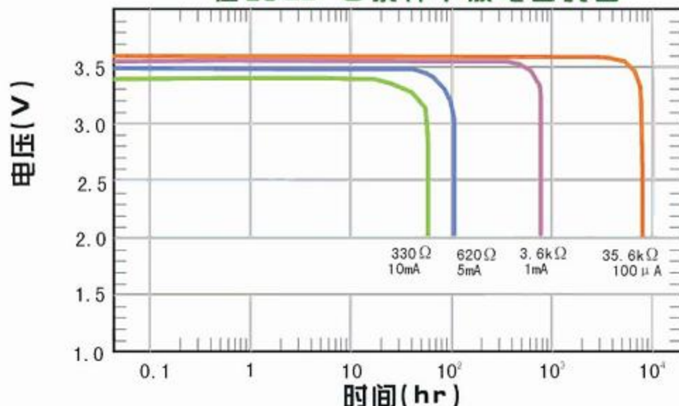
在不同电流,温度条件下容量曲线图
