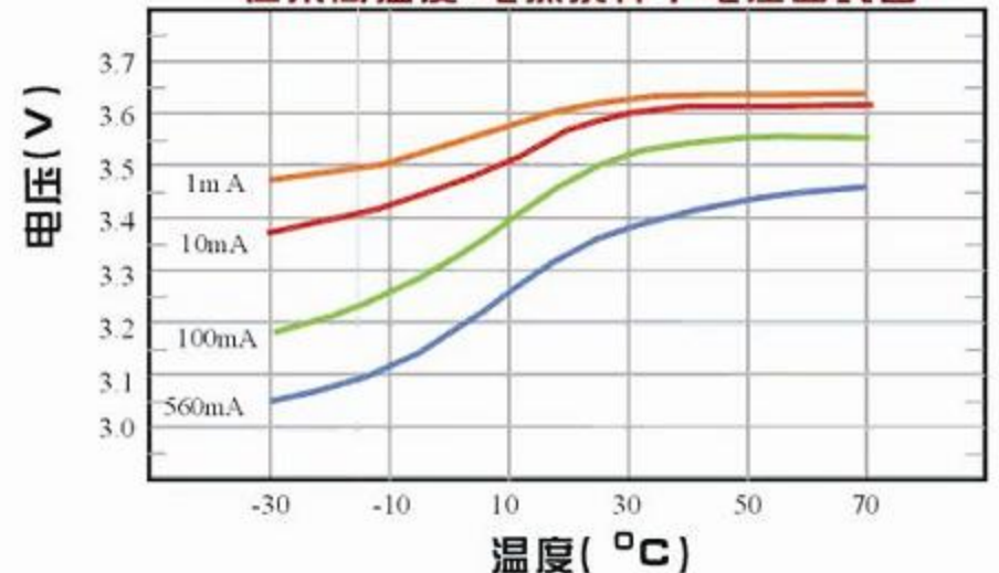
在不同温度,电流条件下电压曲线图
