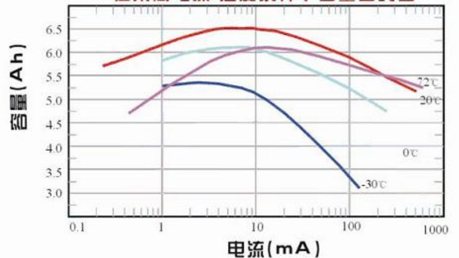
在不同电流,温度条件下容量曲线图
