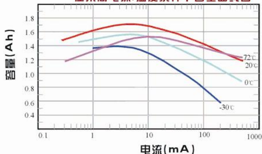
在不同电流,温度条件下容量曲线图
