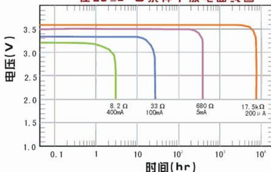
在不同电流,温度条件下容量曲线图
