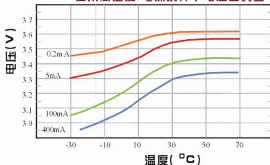
在不同温度,电流条件下电压曲线图
