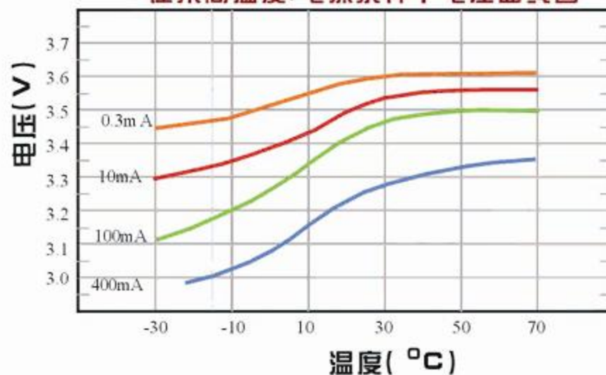
在不同温度,电流条件下电压曲线图
