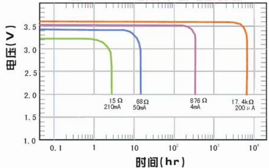
在不同电流,温度条件下容量曲线图
